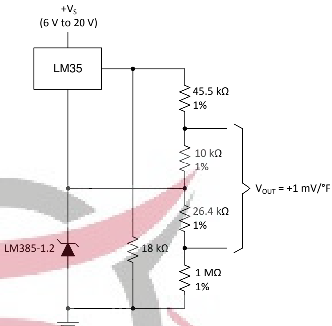
Figure 21. Fahrenheit Thermometer
